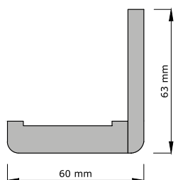
Rozšiřující úhelník pro nastavitelnou zárubeň Rozšiřujúci uholník do nastaviteľnej zárubne
