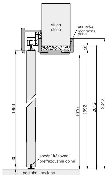
S KONSTRUKCÍ - TUNEL SO ZABUDOVÁNÍM PUZDRA
