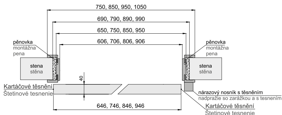
S KONSTRUKCÍ - TUNEL SO ZABUDOVÁNÍM PUZDRA
