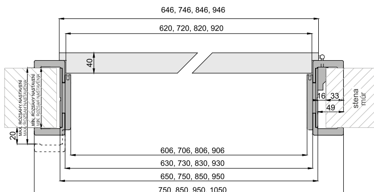
Rozšiřující úhelník pro nastavitelnou zárubeň Rozšiřujúci uholník do nastaviteľnej zárubne
